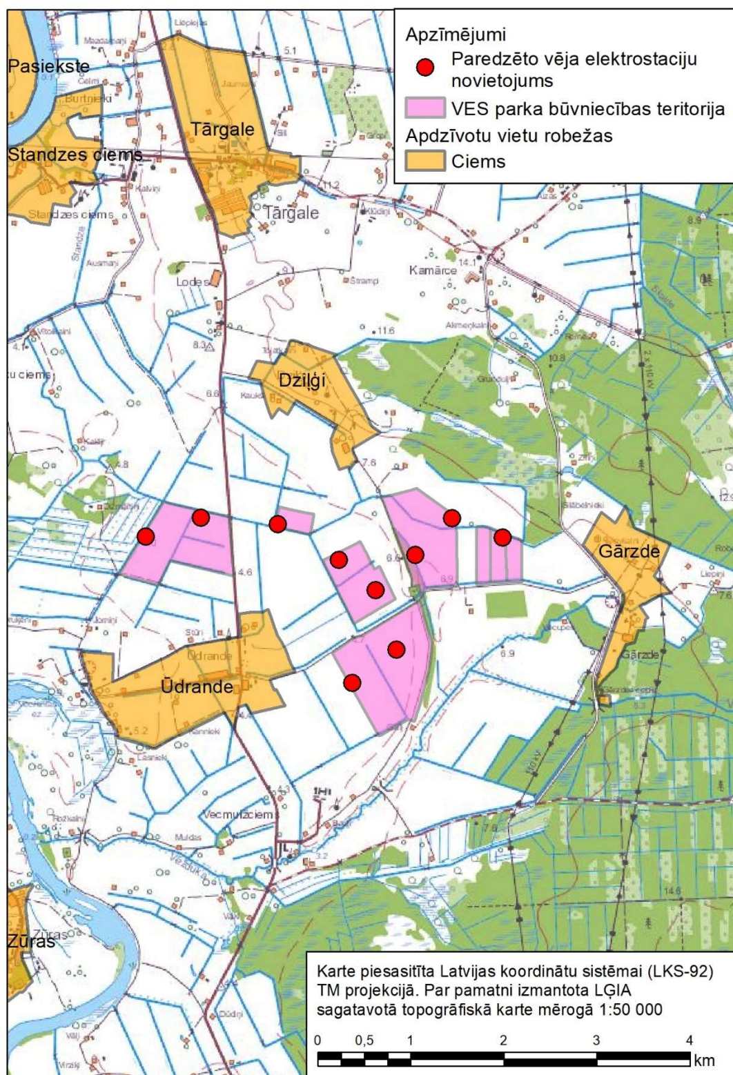
1. attēls. Plānotā vēja elektrostaciju parka „TVE” novietojums
